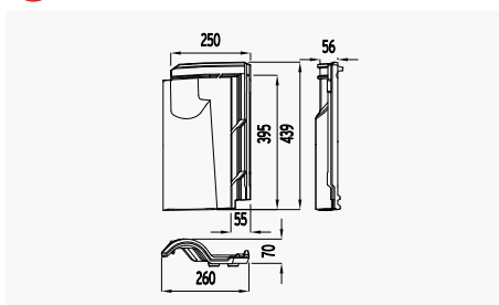
33 Chatière TB-12
