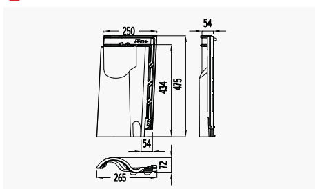
25 Chatière TBS+
