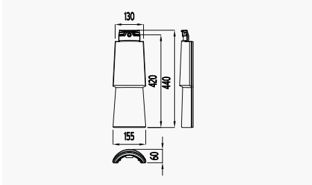
40 Demi-tuile TB-4 / Decocurva Couvrante TB-4 B: Ligne d'égout (Decocurva Couvrante TB-4)
