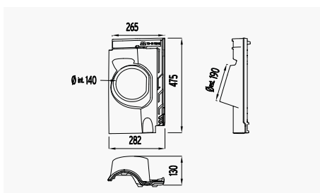
26 Tuile à Douille TB-10 Tech d.140
