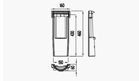
41 Decocurva Courante TB-4
