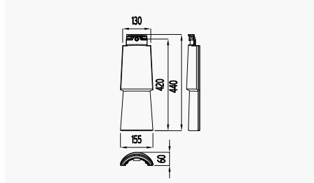
40 Demi-tuile TB-4 / Decocurva Couvrante TB-4 A: Finition latérale droite (Demi-tuile TB-4)
