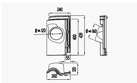
30 Tuile à Douille TB-12 d.140
