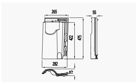
29 Chatière TB-10 Tech
