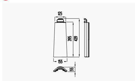
31 Demi-tuile TB-12
