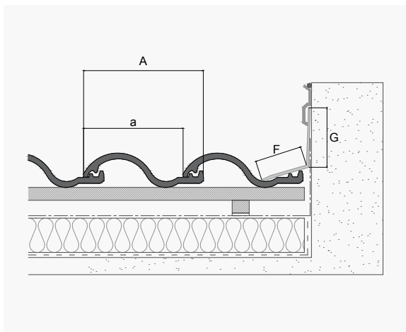
RENCONTRE SUPÉRIEURE
