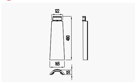
23 Demi-tuile TBS+
