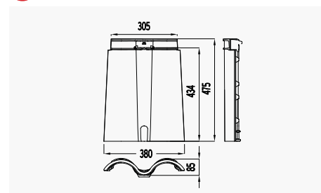
24 Tuile et demie TBS+
