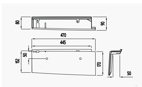
14 Rive à Rabat Gauche
