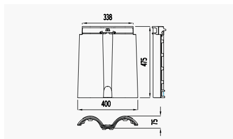
28 Tuile et Demie TB-10 Tech
